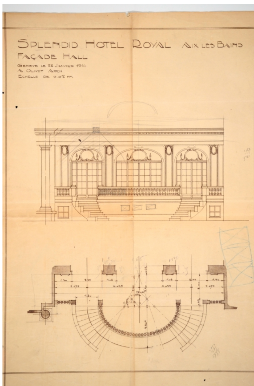
Coupe et élévation de la façade du hall
