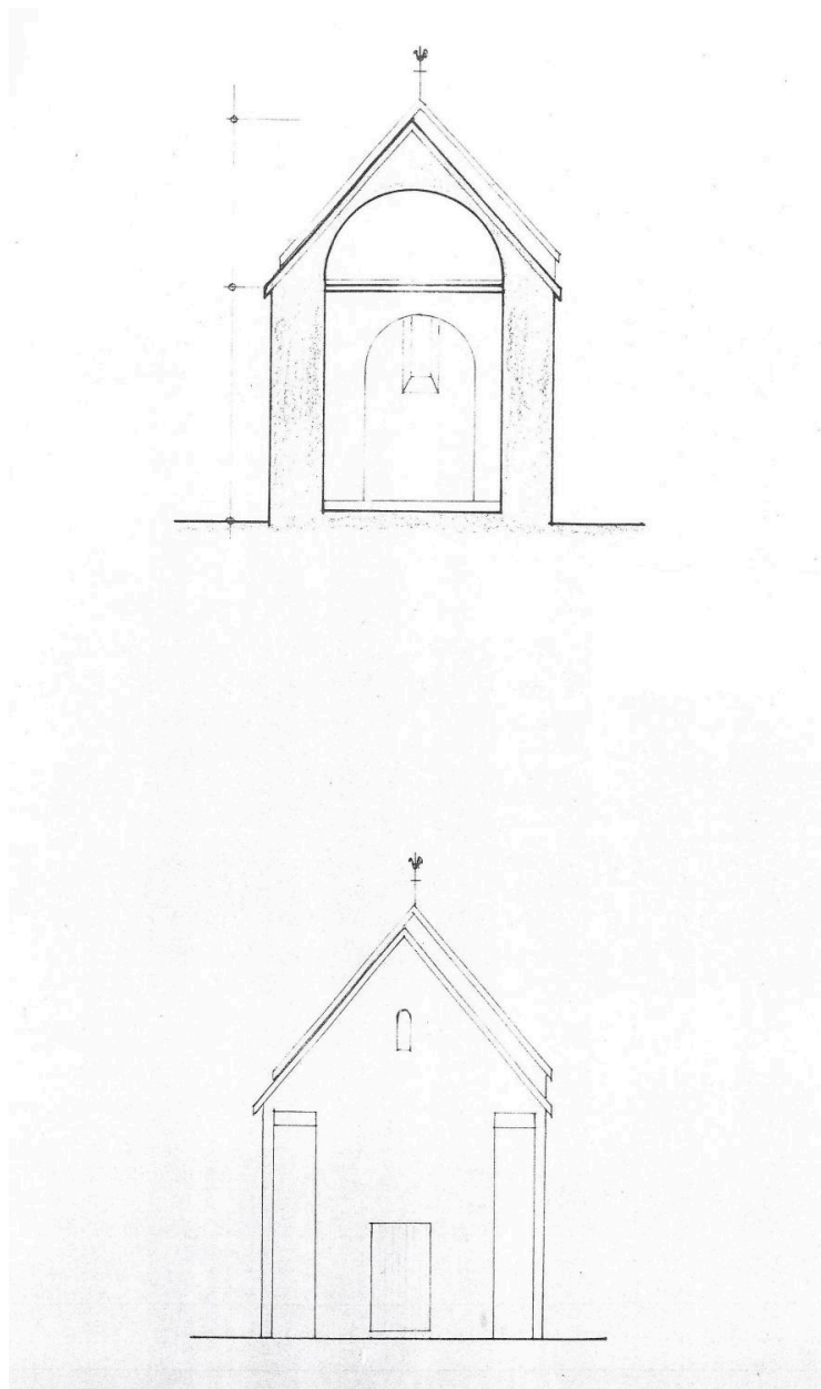
Chapelle : relevé de la façade occidentale et coupe sur le chœur, Agence des Bâtiments de France, Moulins, 1977.
