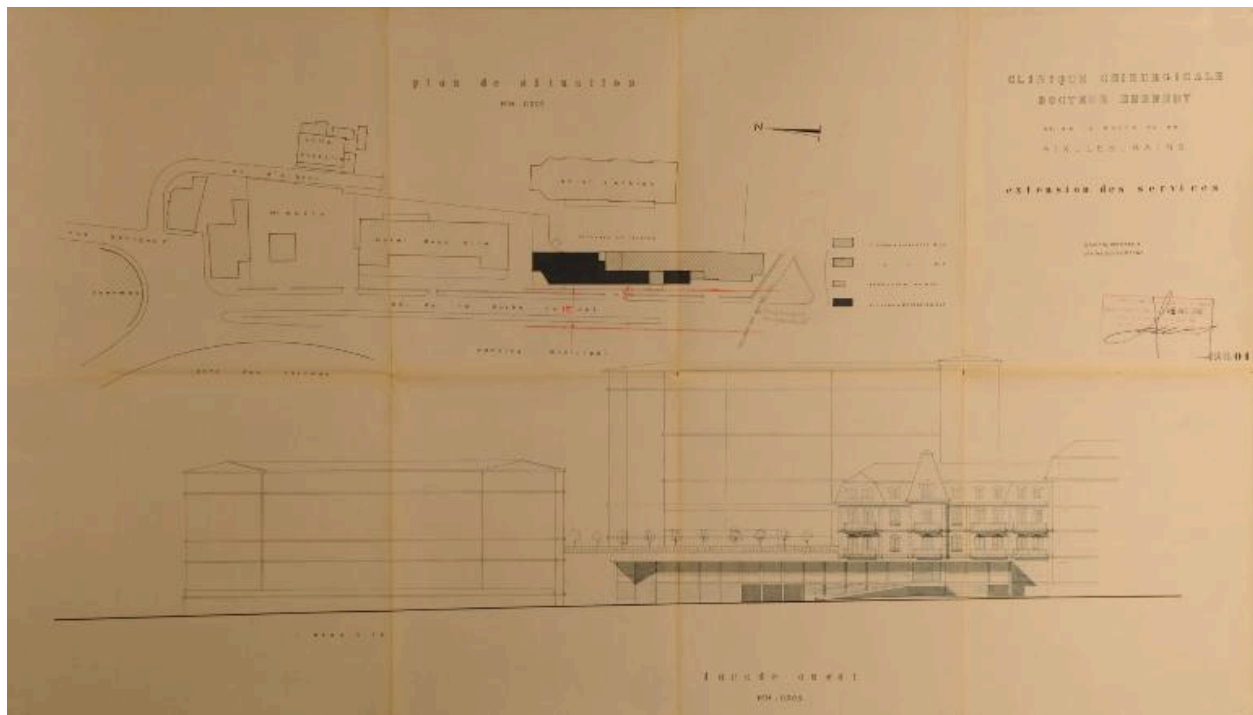
Plan de situation et élévation ouest, extension de 1966
