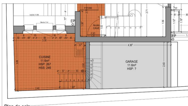
Plan de sols Ech:1/50ème
