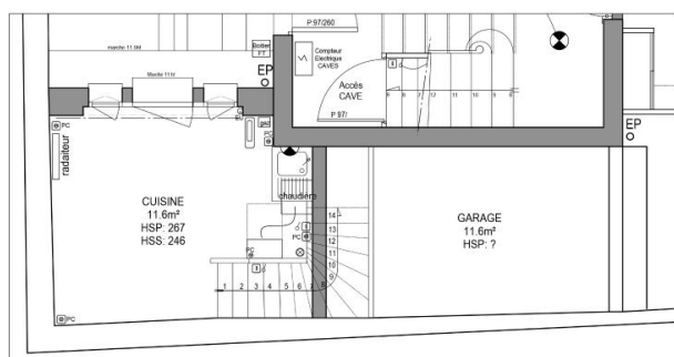
Plan électrique Ech:1/50ème
