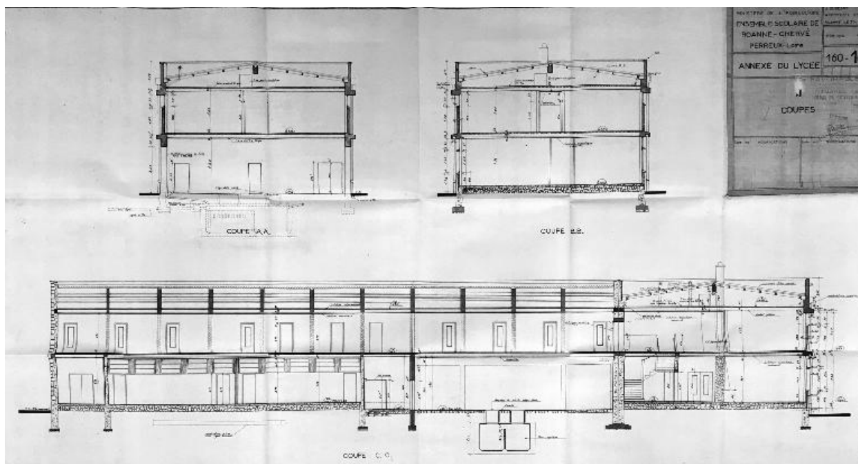
Bâtiment J : coupes, 1965 (AD Loire 690 VT 20)
