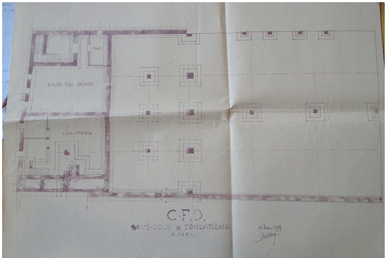
Plan masse de usine des soieries MM Coudurier Fructus et Descher, 1929 (ACL : 344W 845)
