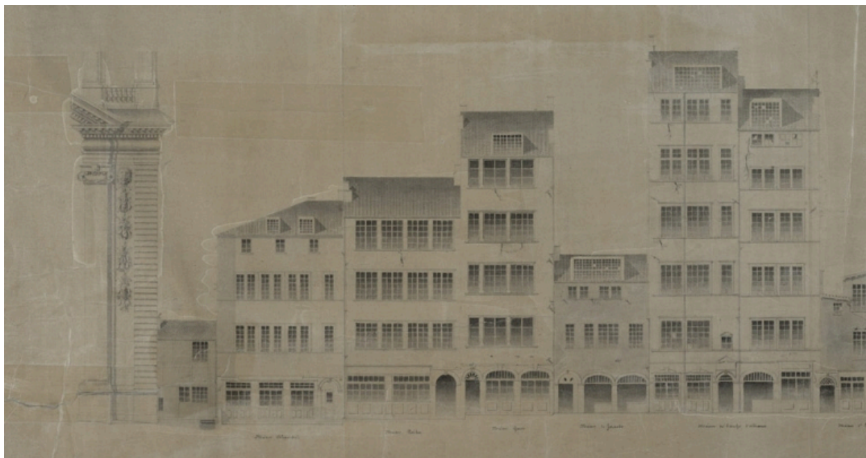
Maisons à démolir rue Bourchanin : détail nord du relevé
