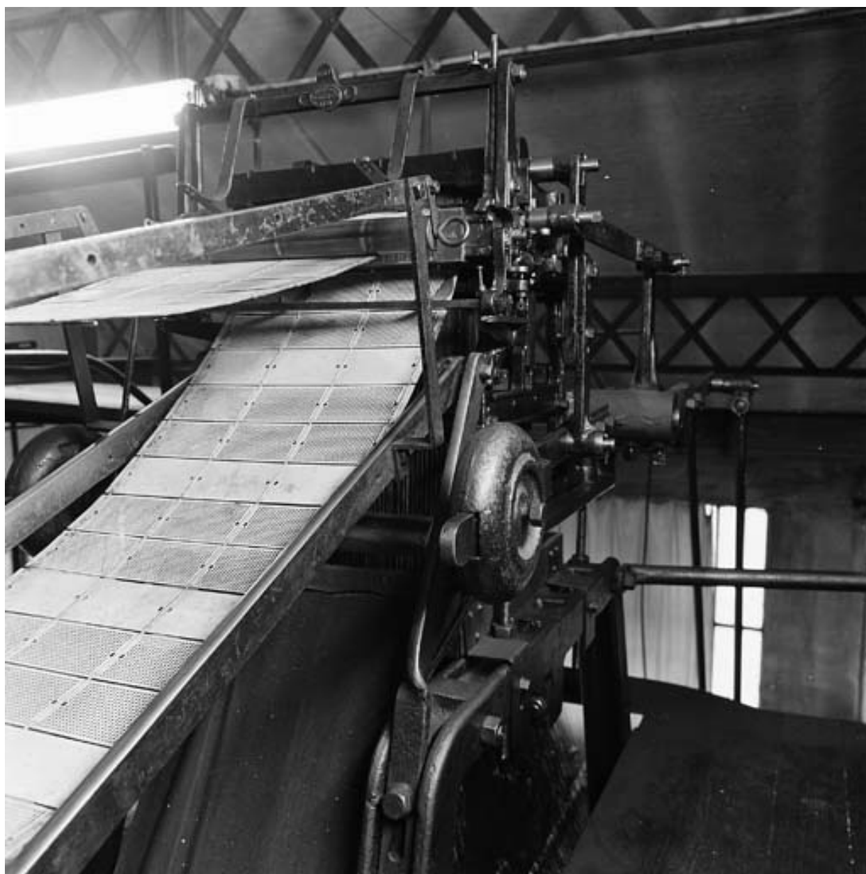
Détail passage carton perforé
