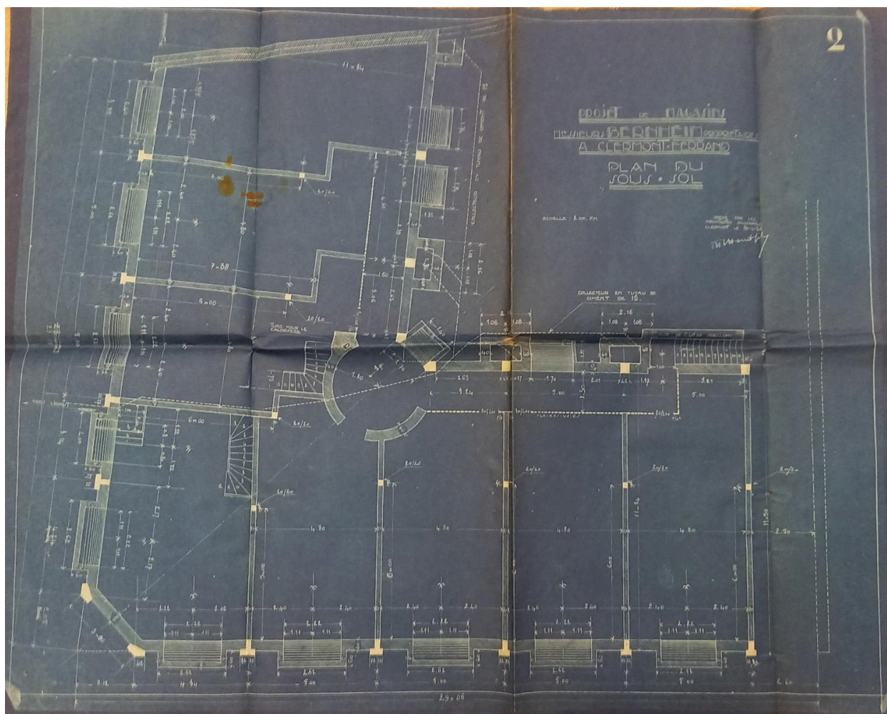
Plan du sous-sol, 21 avenue Charras
