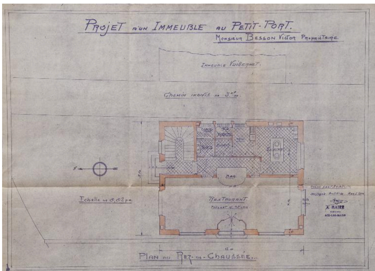
Hôtel Besson, 1934 : plan du rez-de-chaussée
