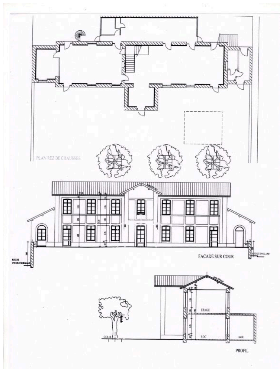
Plan, coupe, élévation, 2e moitié 20e siècle (AC Montbrison, bureau de'études).
