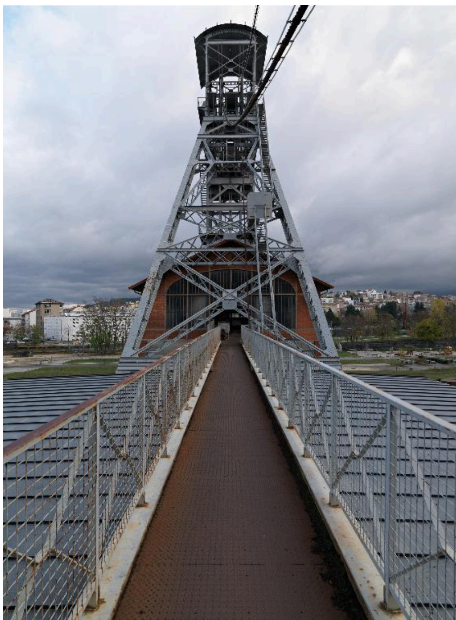
Passerelle d'accès au chevalement, vue ouest
