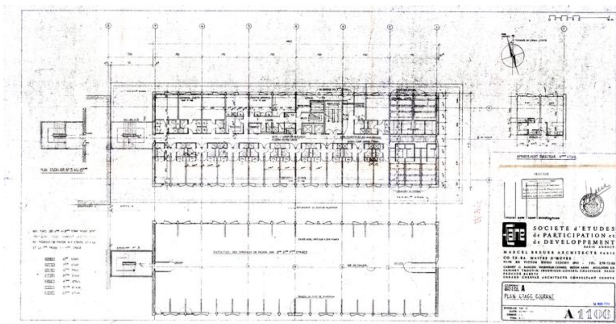
Hôtel A. Plan d'un étage courant. Marcel Breuer architecte, 26 août 1968 (AC Arâches-la-Frasse)
