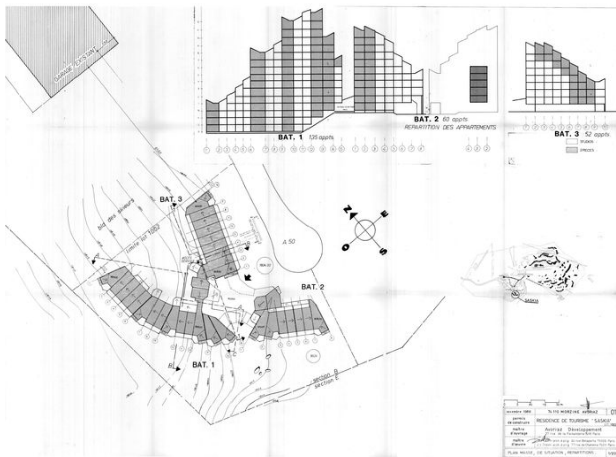
Plan masse, de situation, répartitions / J. Labro, J. J. Orzoni, novembre 1986 (AC Morzine)
