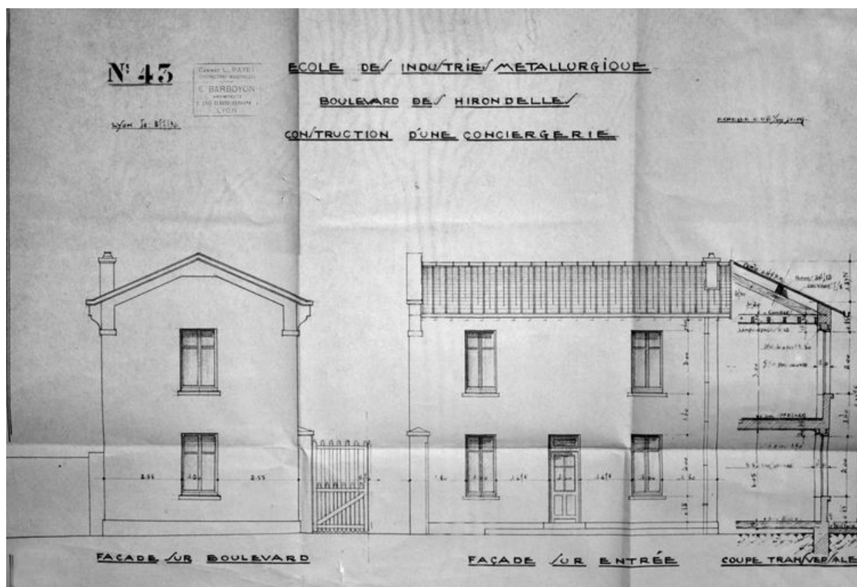
Façades et coupe transversale de la conciergerie (Barboyon), 1930
