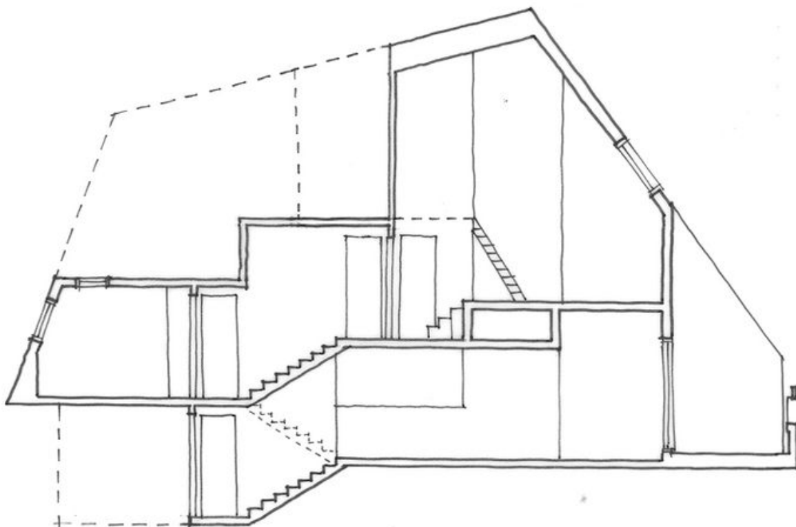
Mélèze I. Appartement 45. Coupe. Relevé schématique
