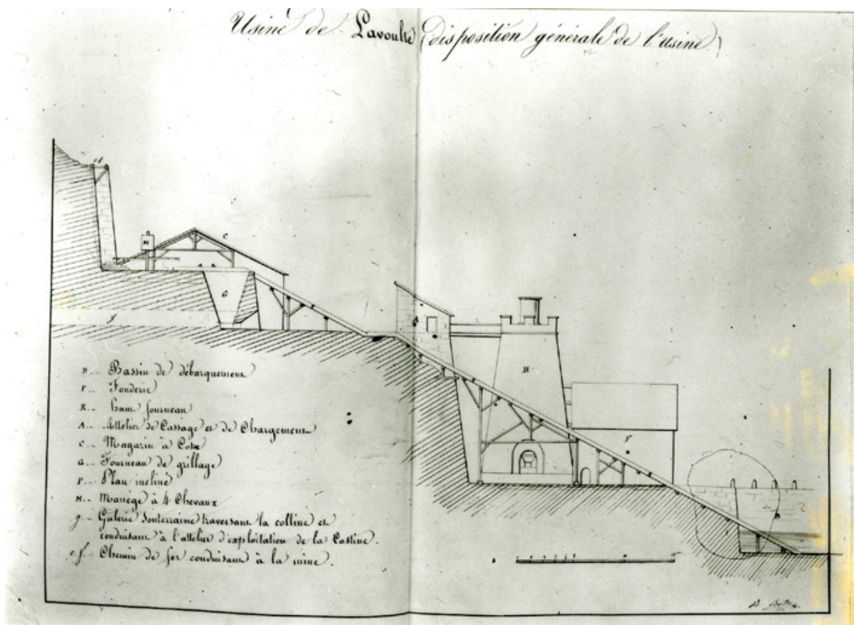
Coupe représentant la disposition générale du site (vers 1848)
