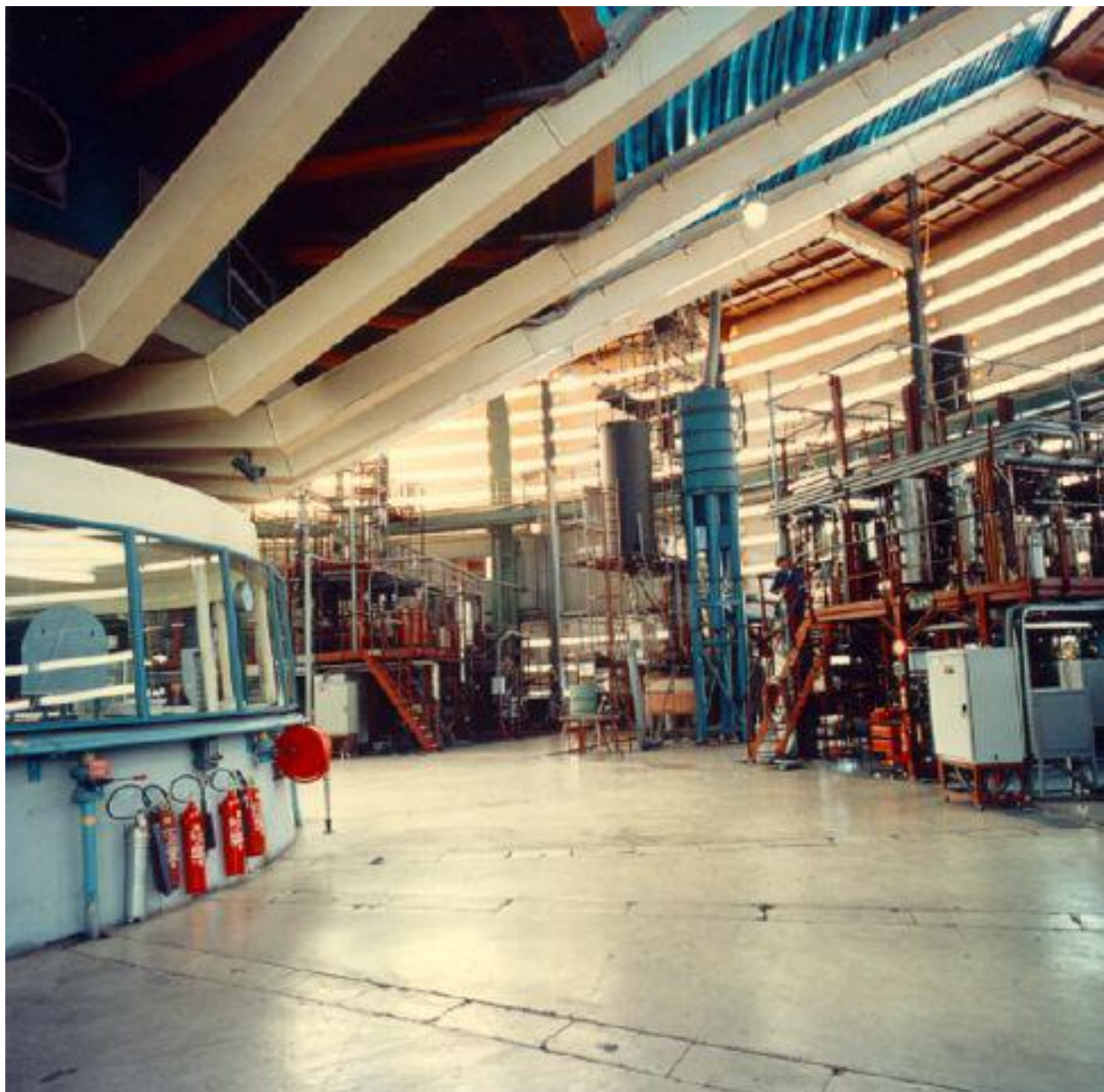
Hall des Unités pilotes à Solaize (vue d'intérieur)
