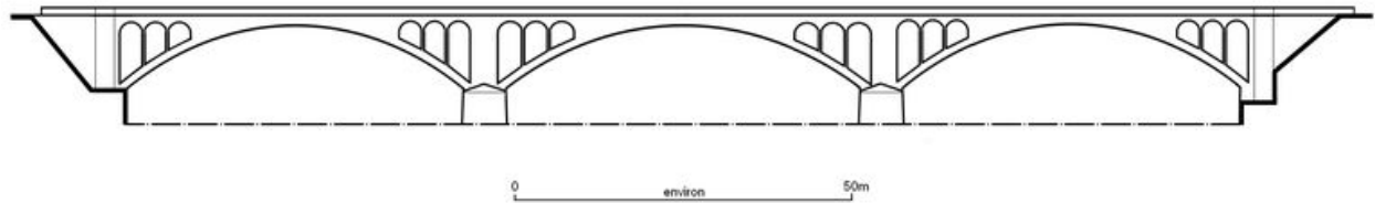
Elévation aval (relevé schématique)
