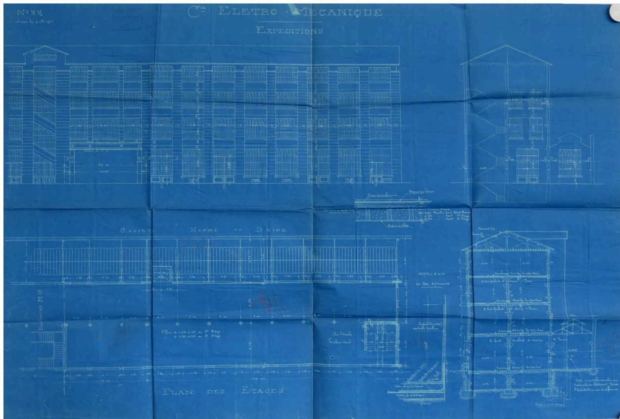
Plan des étages 1918 (AC Lyon314W/593)
