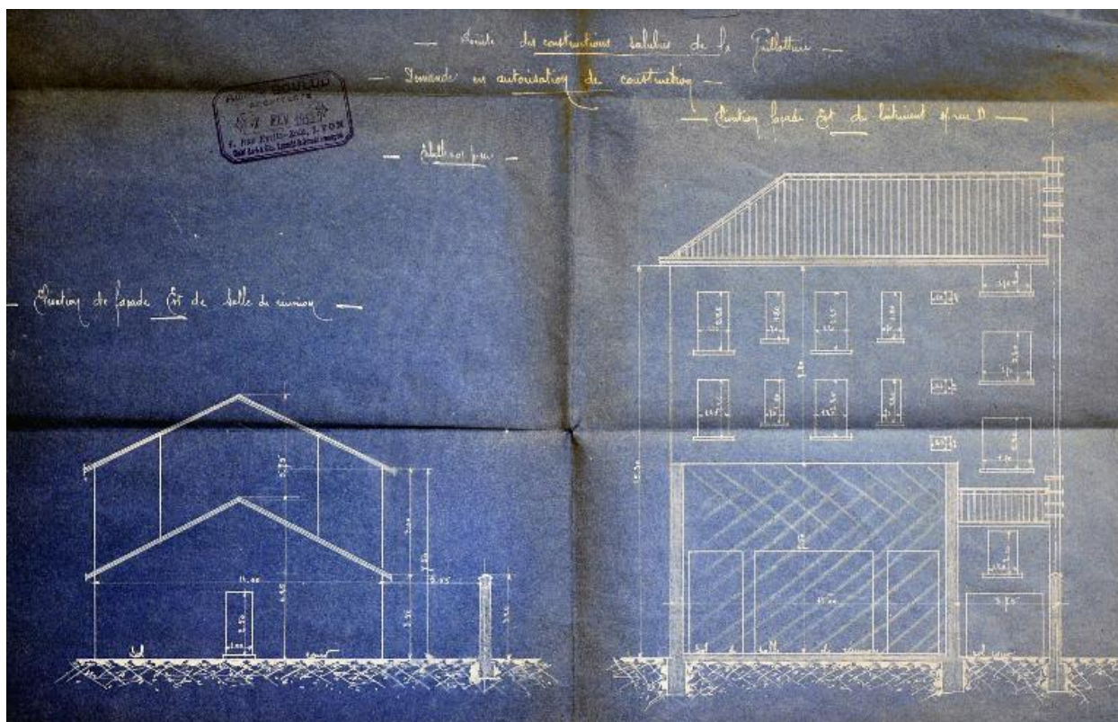
Elévation façade est bâtiment sur rue D (rue Nicolaï) par A. Boulud, 1913 (AC Lyon)
