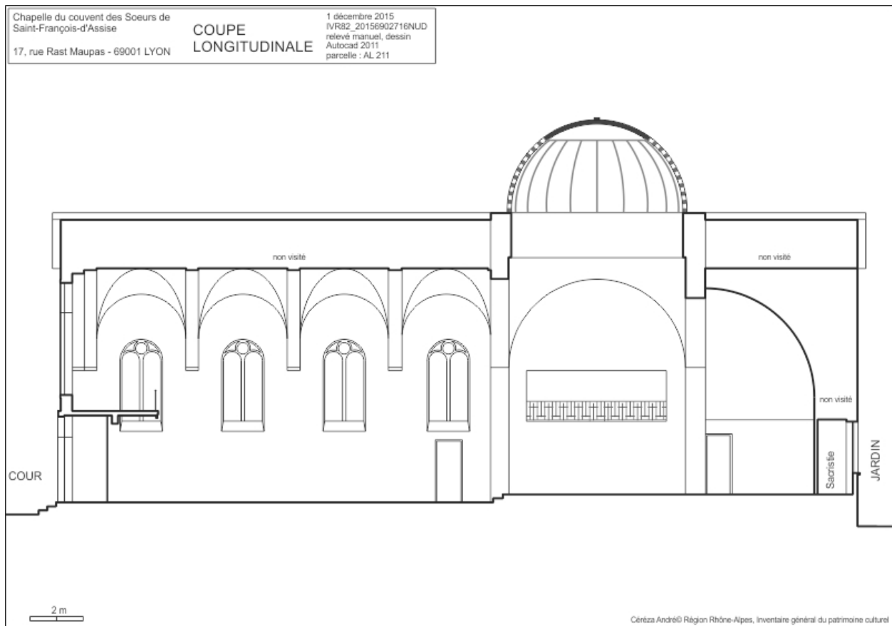
Coupe longitudinale
