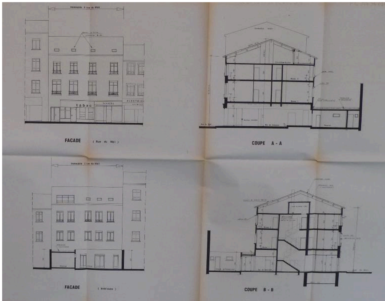
Elévations et coupes de l'immeuble après la restructuration de 1994 (Arch. Mun. Lyon, 1797 W 116 : Permis de construire et de démolir, 1993)
