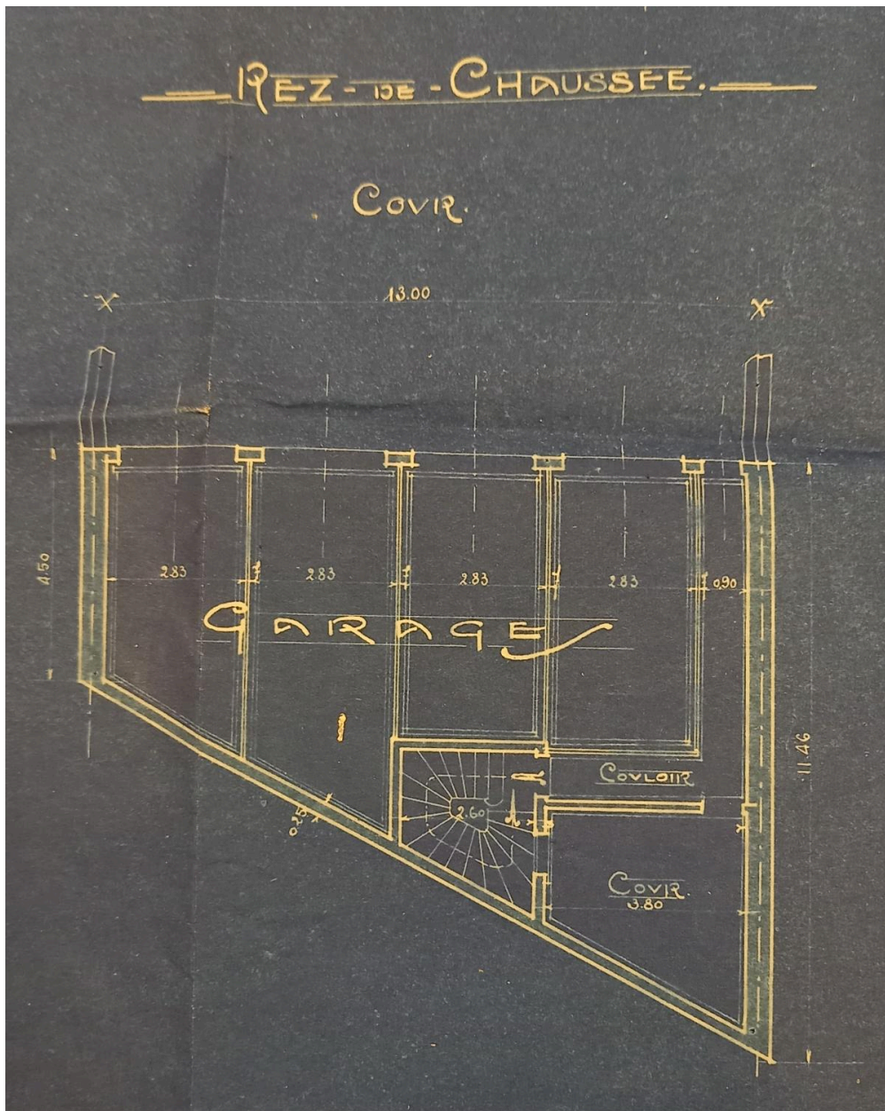
Plan du rez-de-chaussée de la maison de fond de parcelle
