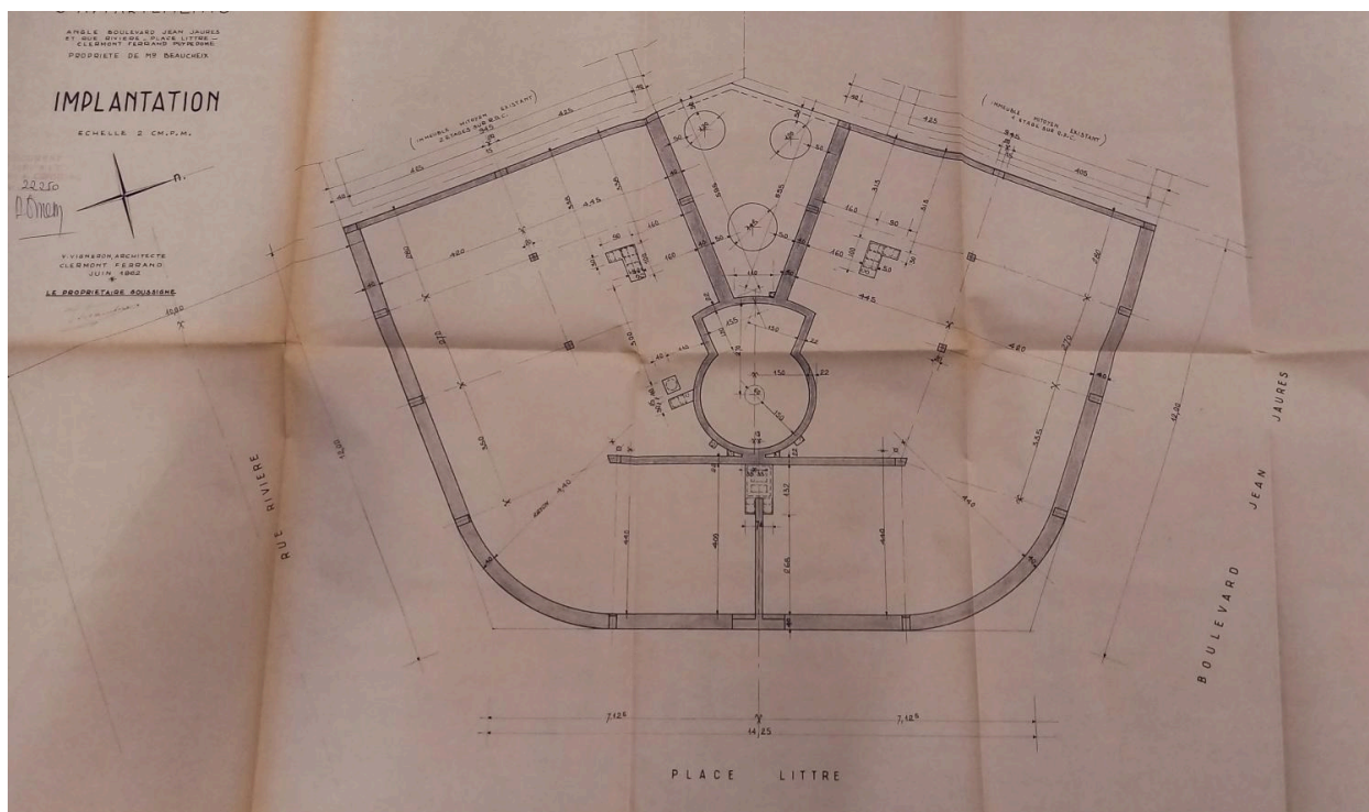
Plan d'implantation
