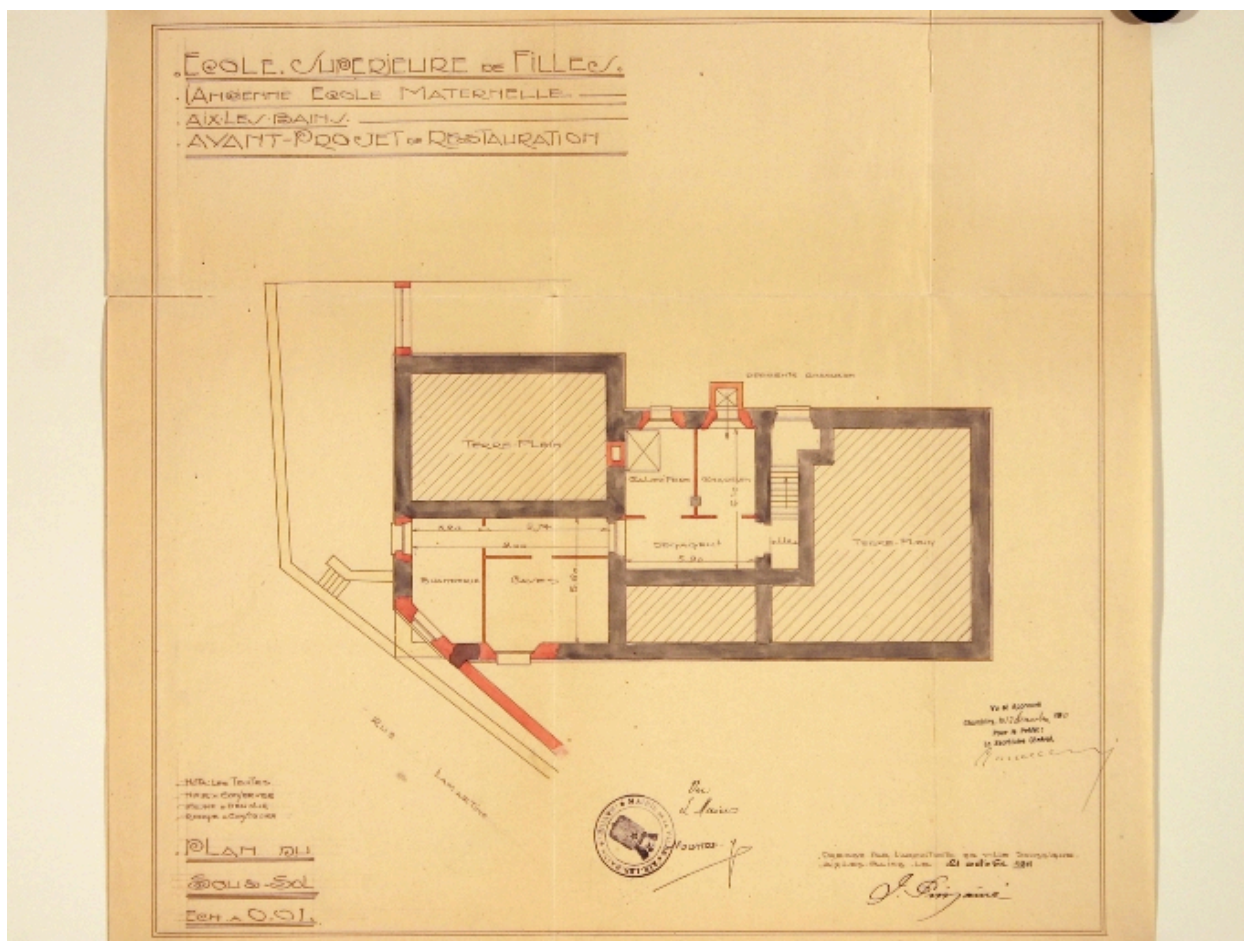
Plan du sous-sol, 1911
