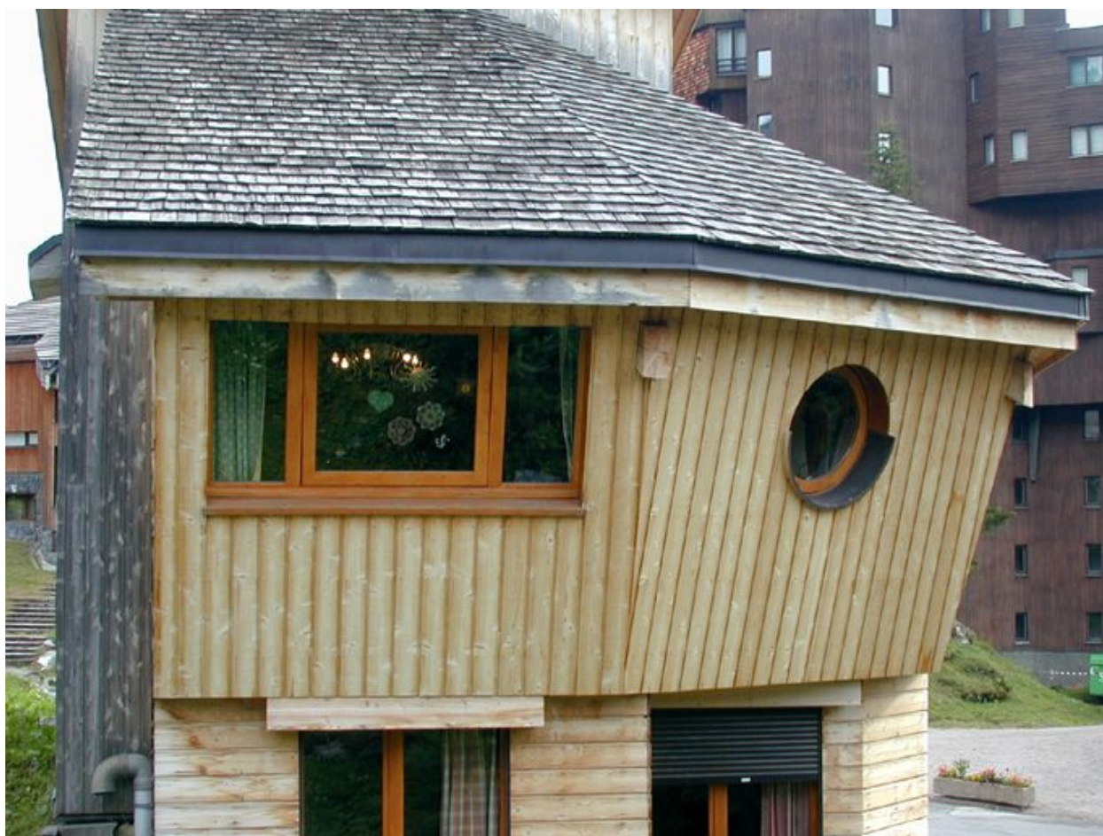
Détail de l'élévation nord
