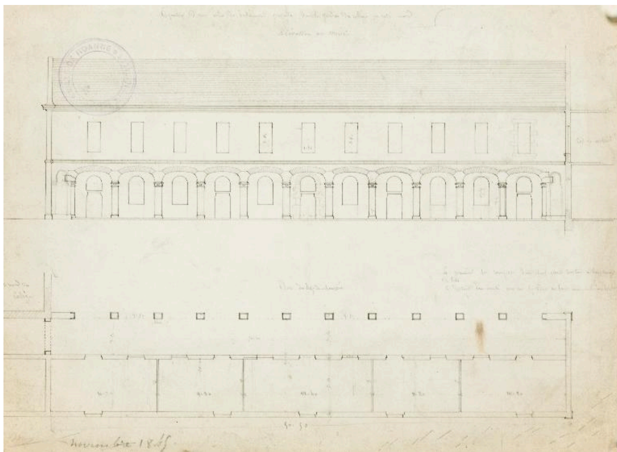
Élévation et plan d'un bâtiment sur galerie et étage. (1845)
