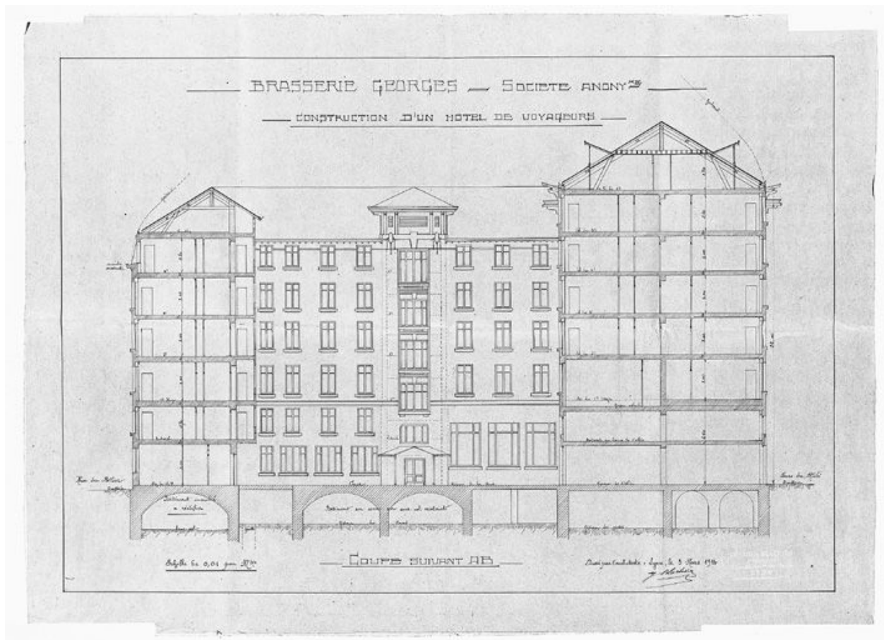
Coupe longitudinale
