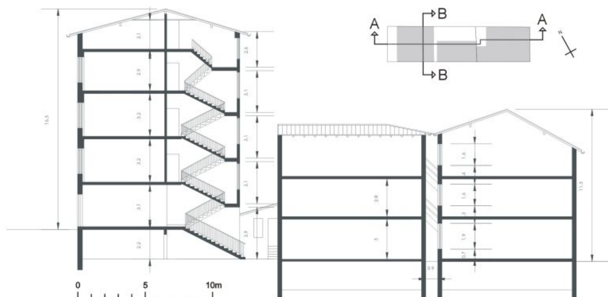
Coupe longitudinale AA, d'après A. Spinoza-Beaurain, architecte, 2001.
