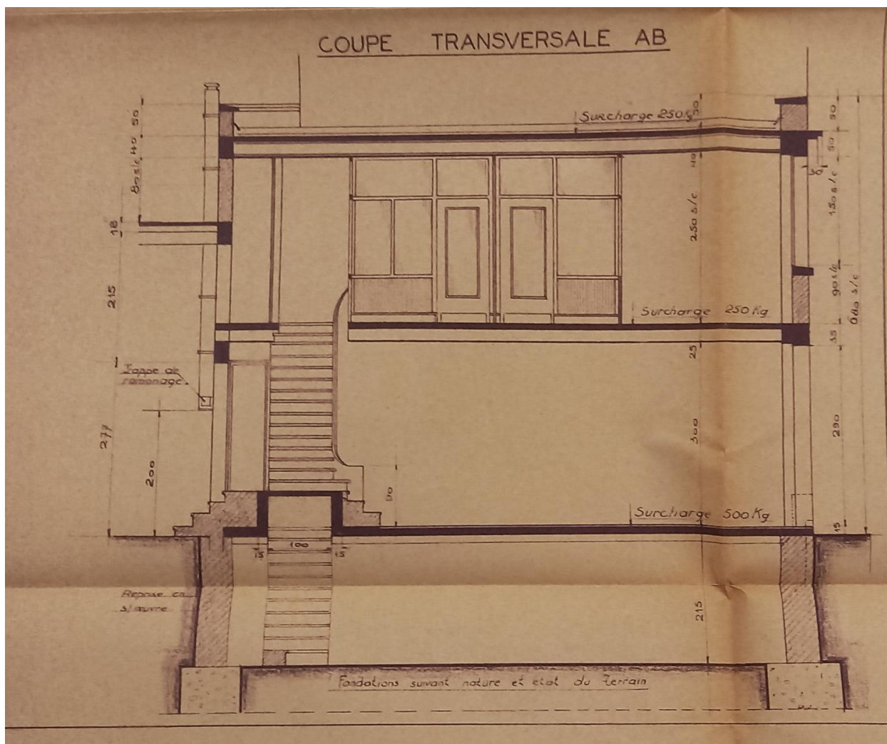
Coupe transversale
