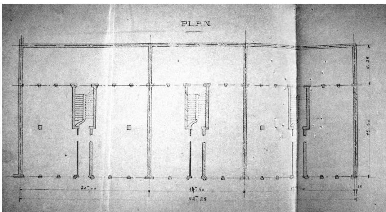
Plan des rez-de-chaussées (AC Lyon, 314 WP 1899)
