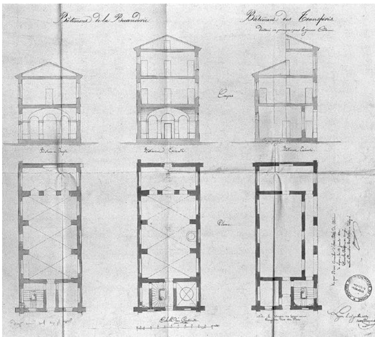
Plans et coupes du bâtiment de la buanderie et du bâtiment des transférés destiné en principe pour les jeunes condamnés, par l'architecte Dumont, 16 juillet 1829. 49 x 61 AD, Rhône. 1 Y 299
