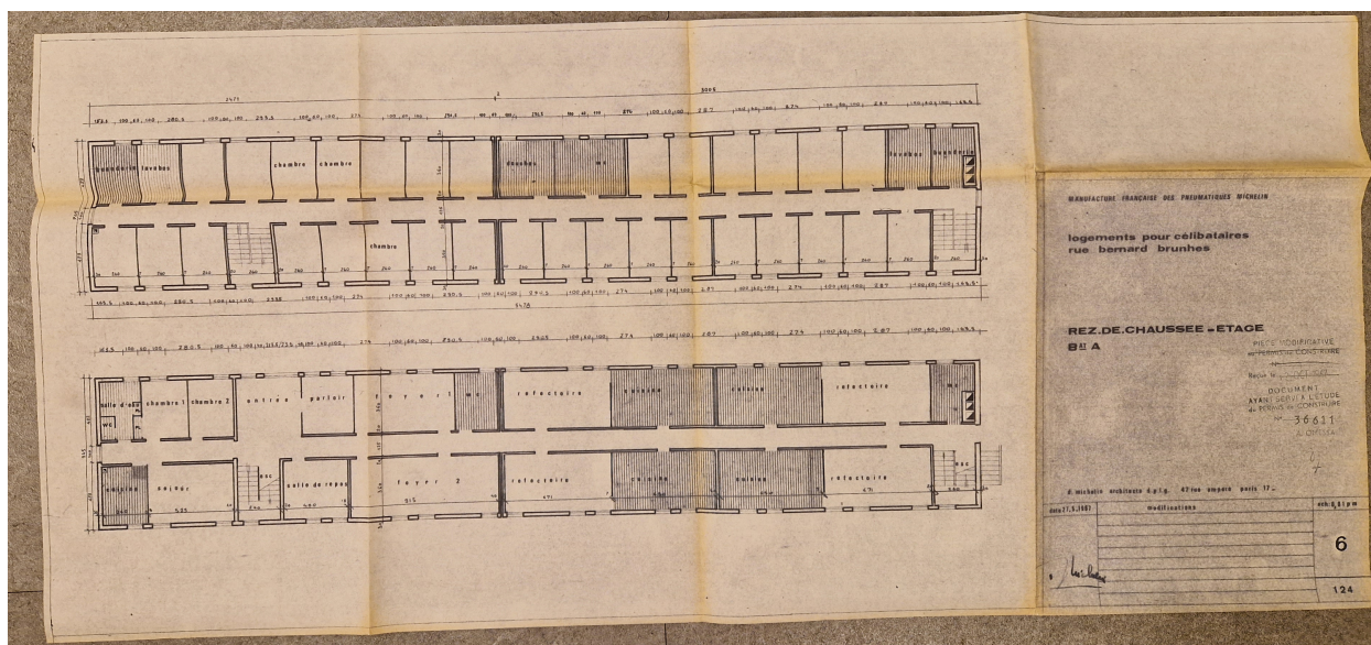
Plans du rez-de-chaussée et de l'étage du bâtiment A de la rue Bernard-Brunhes, par Daniel Michelin, 1967.
