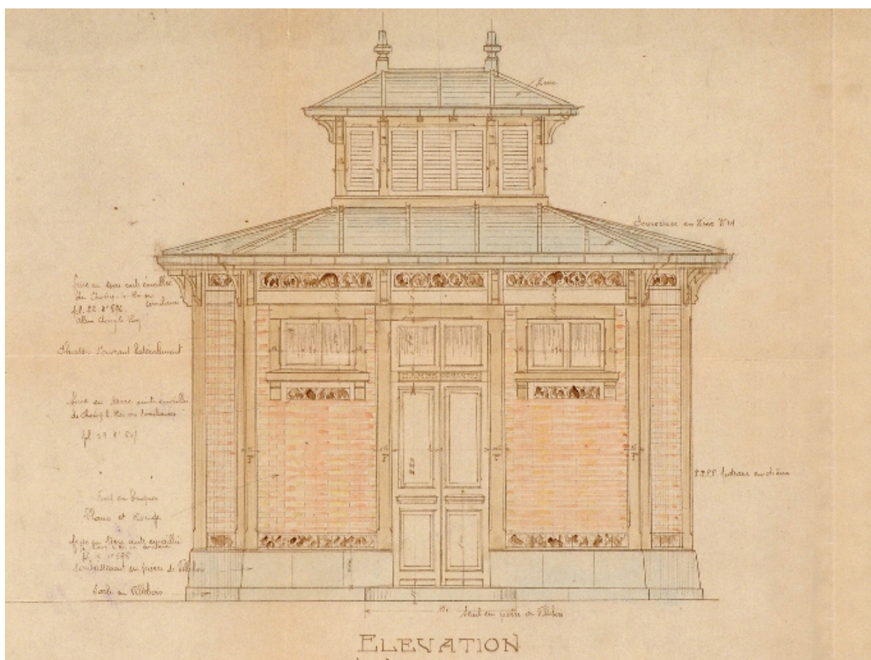
Projet de chalet de nécessité, élévation principale
