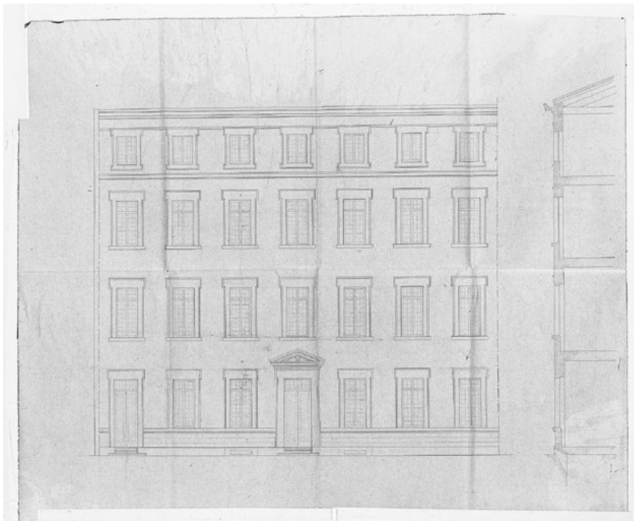
Elévation ouest
