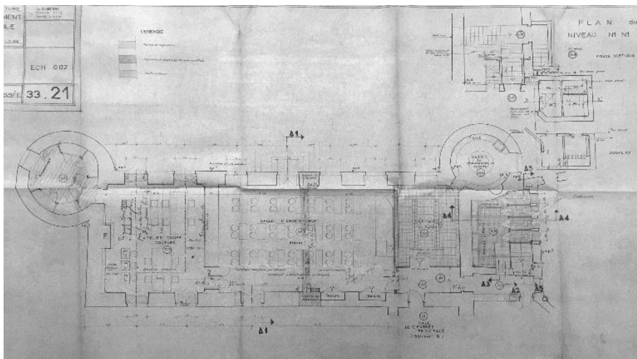
Château, corps de bâtiment A : plan d'exécution, rez-de-chaussée, 1954 (AD Loire, 690 VT 39)
