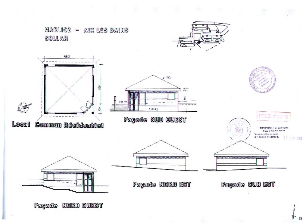
Plan et élévations du local commun
