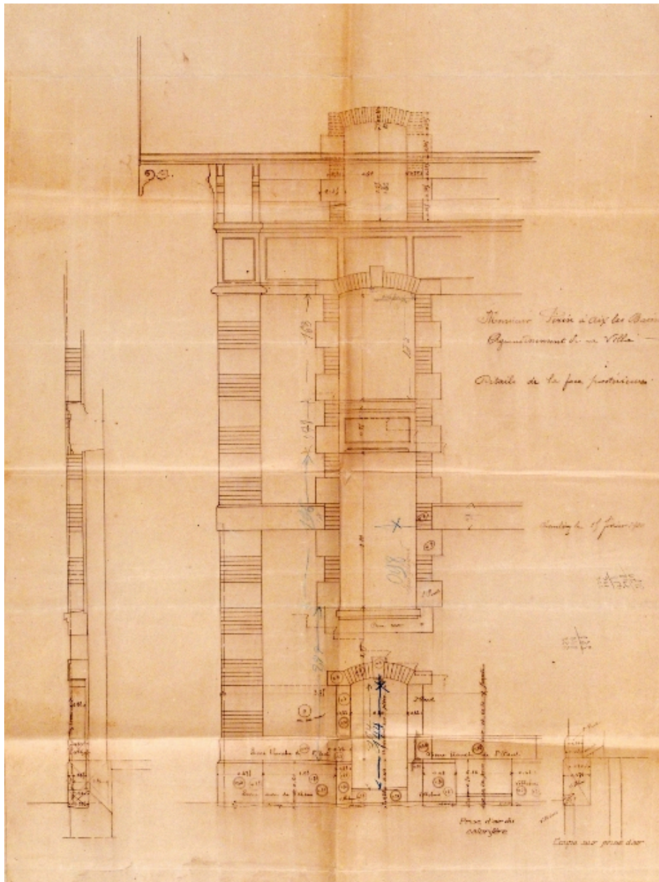
Élévation postérieure, détail d'une travée de baies
