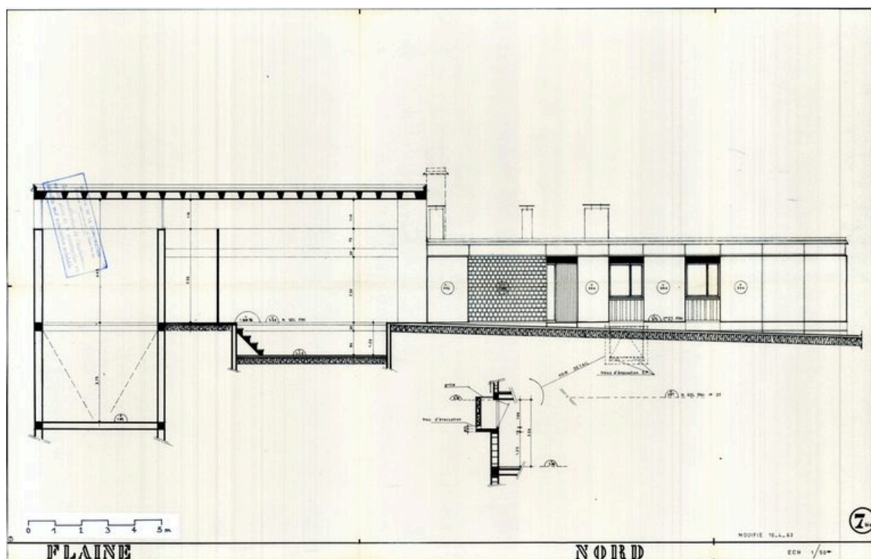
Elévation nord. [Laurent Chappis, Agence Berthe, Chappis, Jomain architectes, 1962]. Modifié le 10 avril 1963 (AC Arâches-la Frasse)
