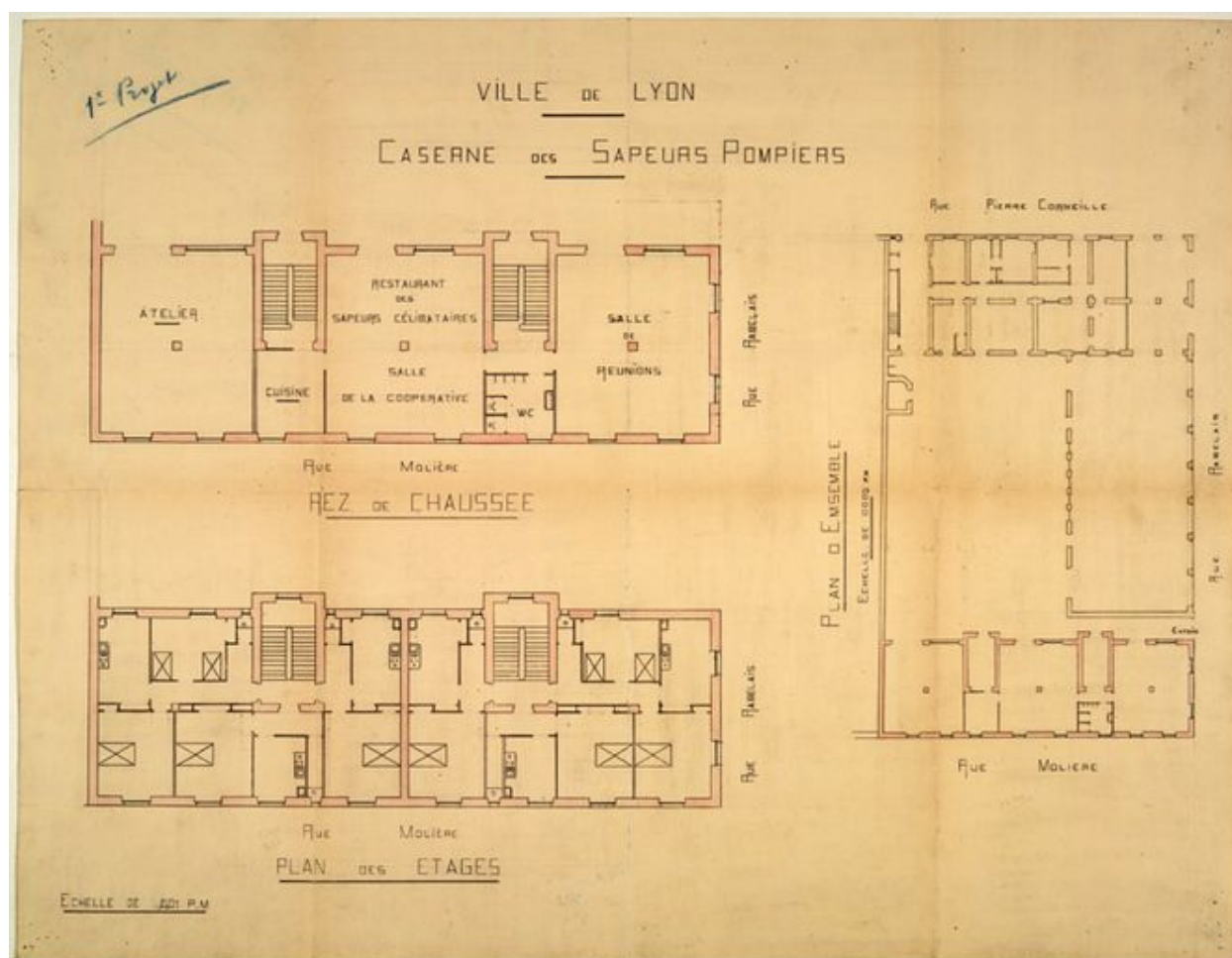
Plan d'ensemble, plan du rez-de-chaussée et plan des étages du premier projet
