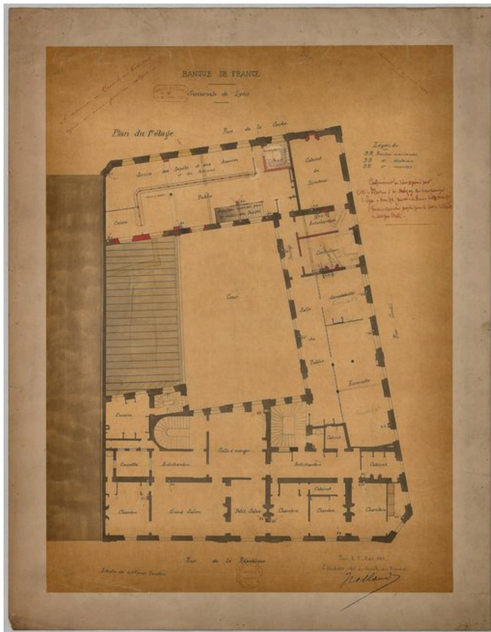
Plan du 1er étage avec les mentions de transformations entraînées par le déplacement du bureau et de la serre des dépôts du 1er étage au rez-de-chaussée (1892) (Banque de France, PHAR, non coté, dessin de JC Merlin).
