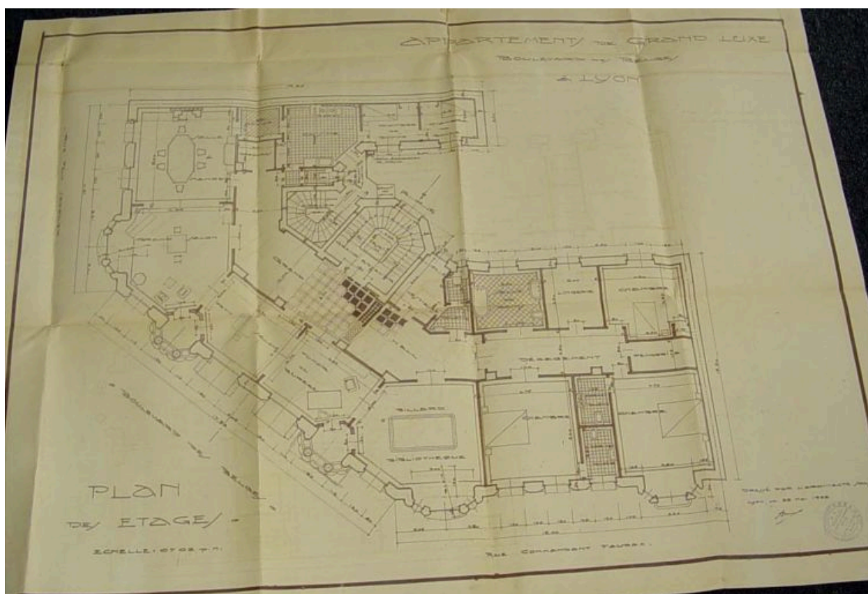
Plan des étages / Bornarel, 1928
