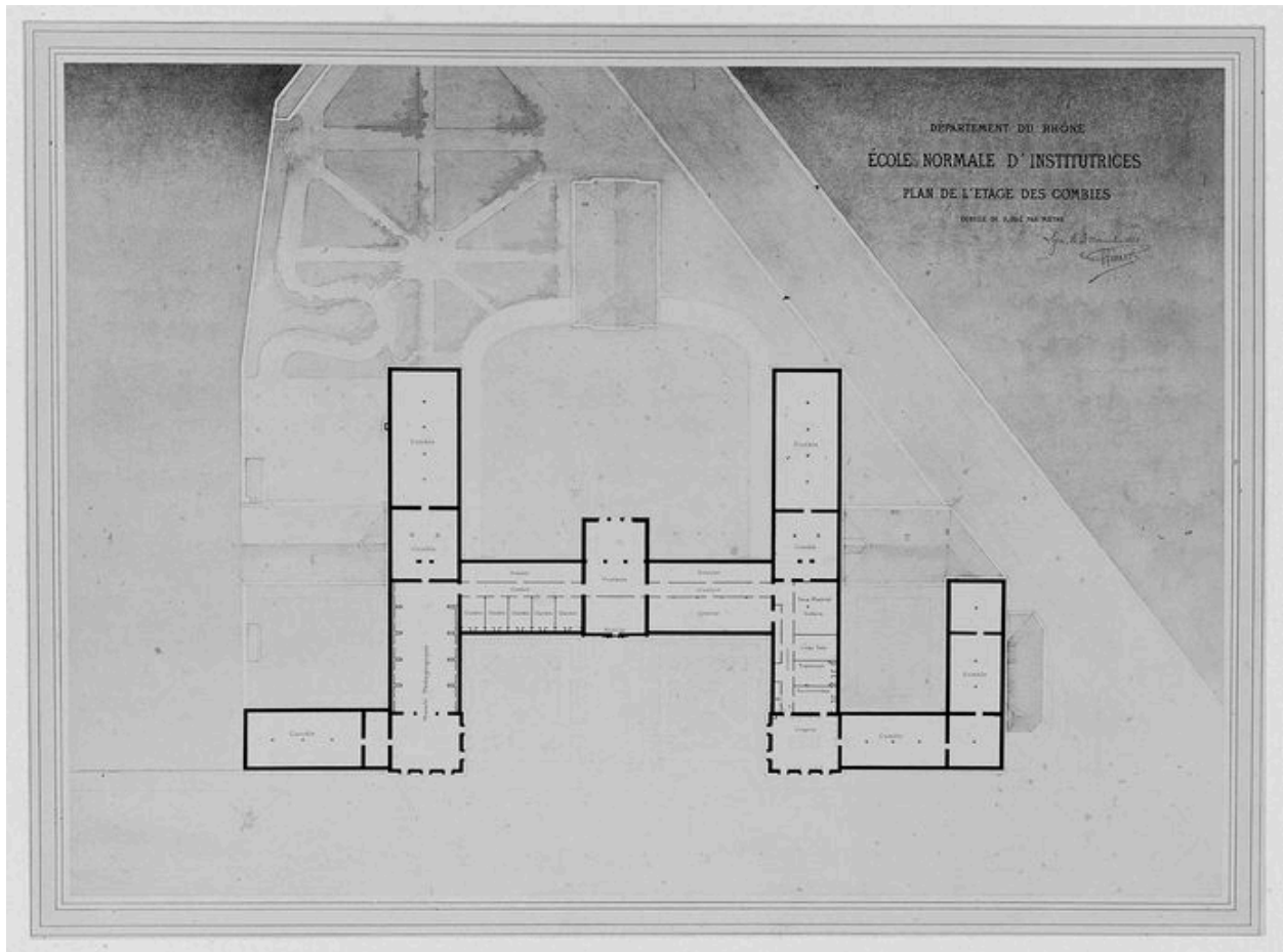
Plan des combles (1888) (Arch. dép. Rhône, 1 T 1267, photographie de Fernique).
