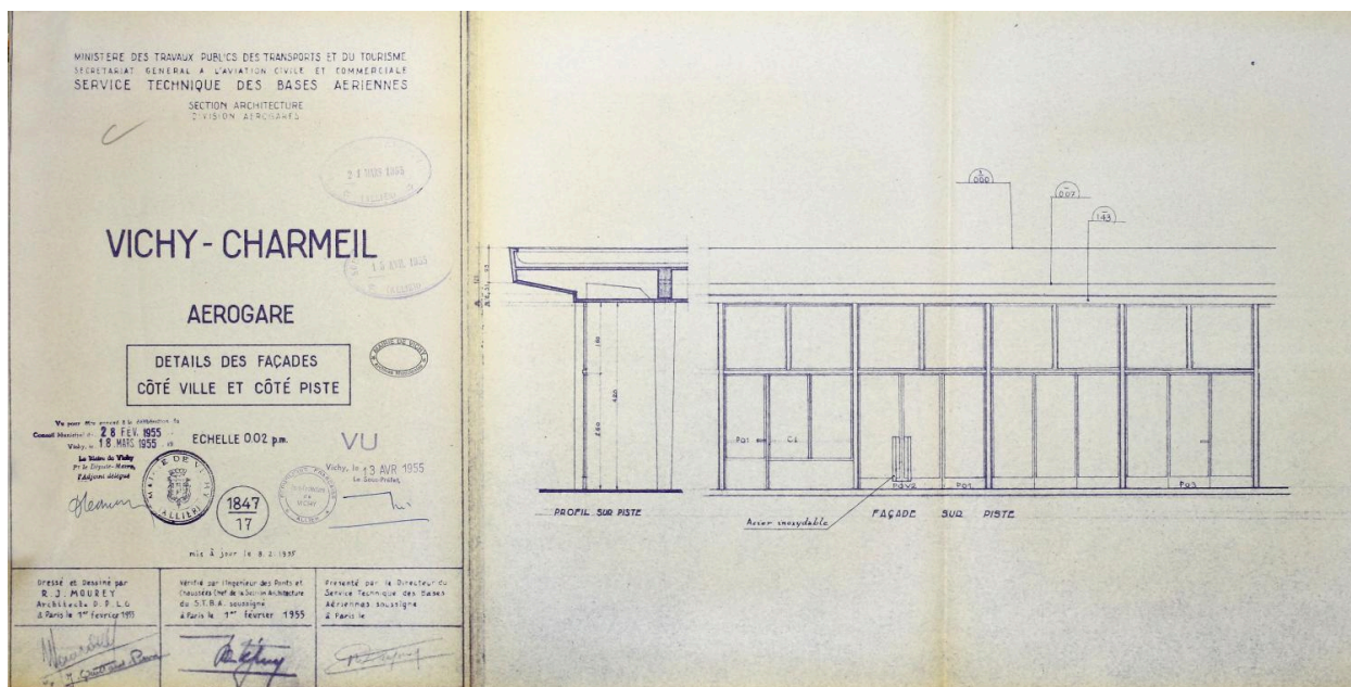
Détail de la façade côté piste (est) de l'aérogare de Vichy-Charmeil, février 1955, Service technique des bases aériennes (Archives municipales de Vichy).
