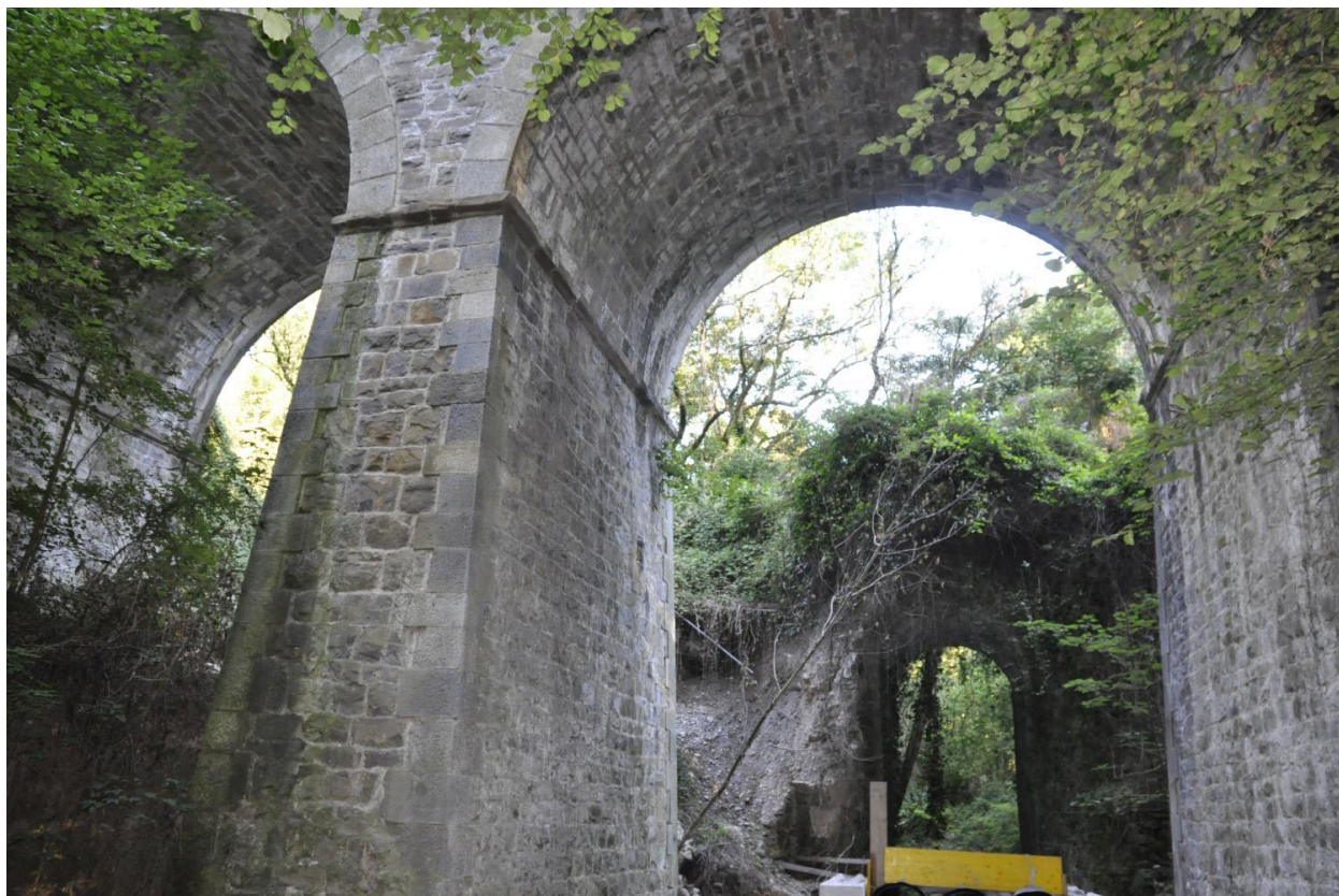
Vue de la face amont du pont vieux prise en amont du viaduc
