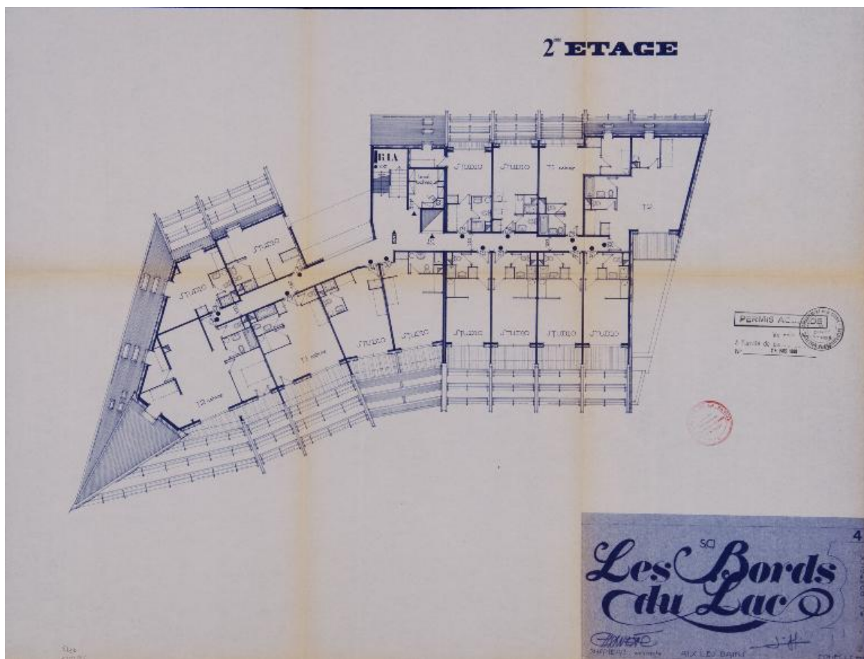
Les Roseaux, 1980 : plan du 2e étage
