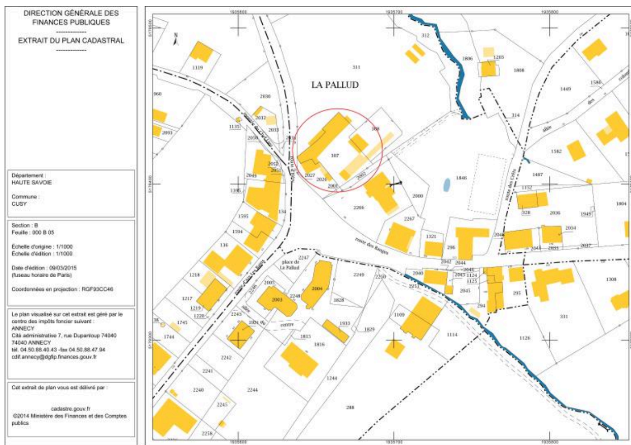
Plan masse de la ferme de la Pallud
