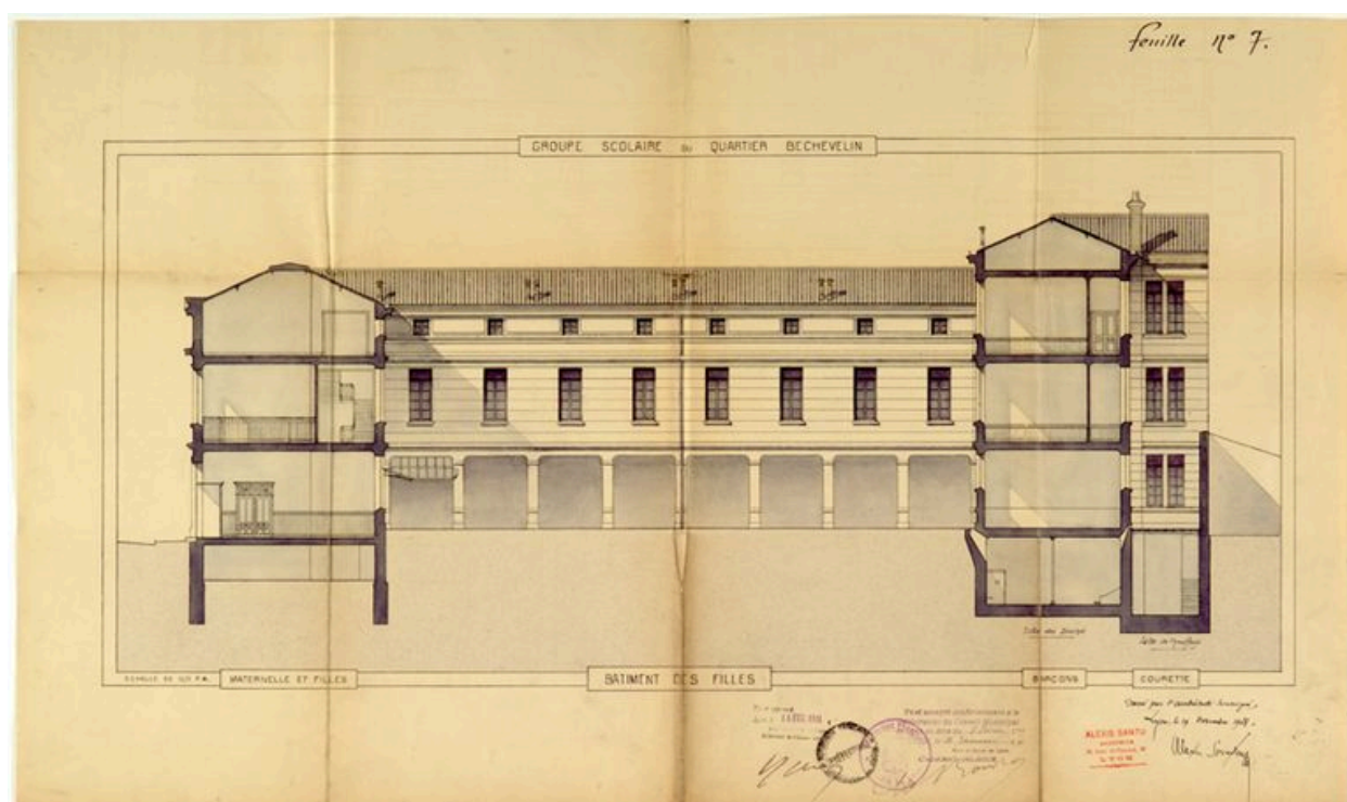
Élévation du bâtiment des filles, 1908 (AC Lyon. 0476 WP 53)
