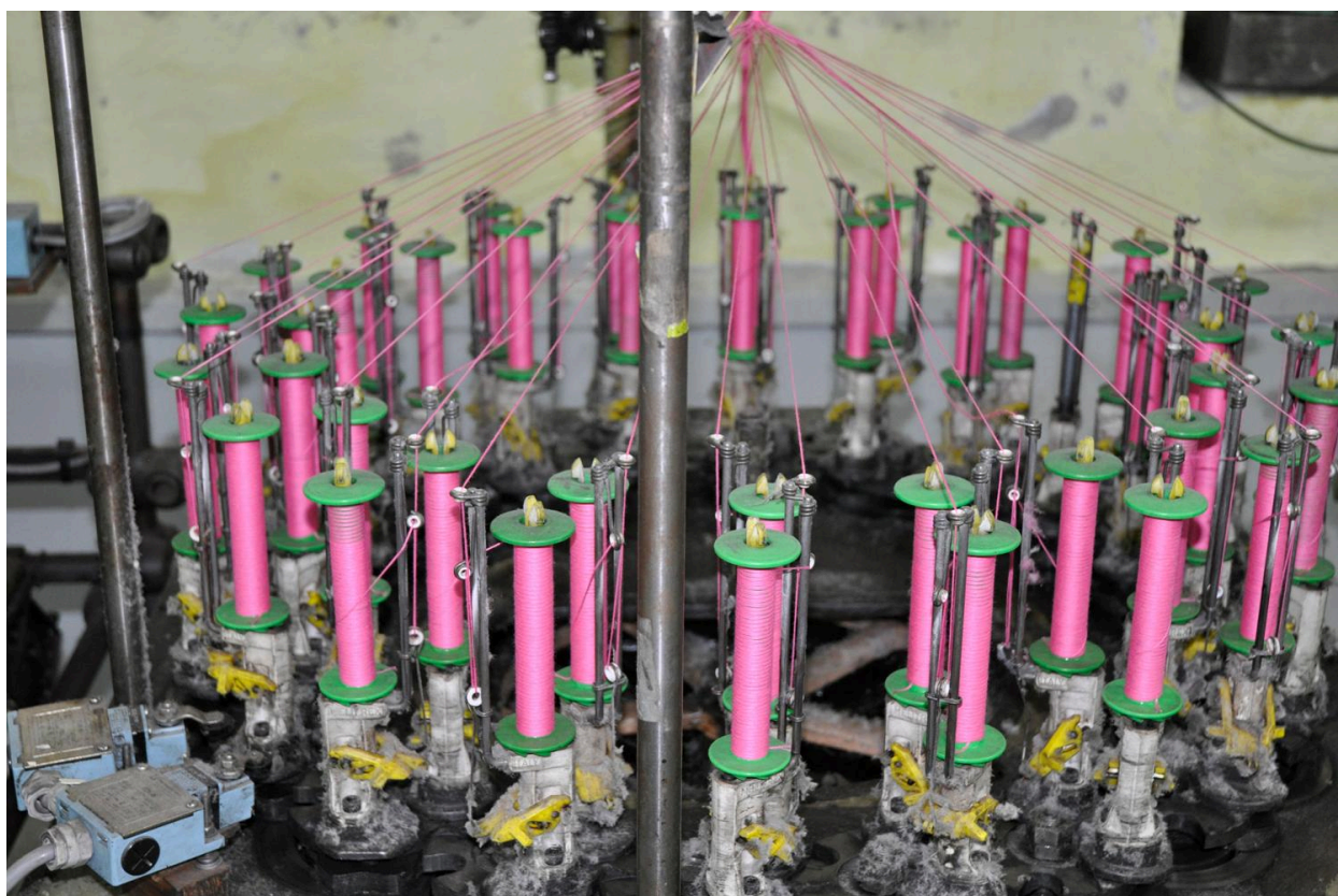
Détail métier à tresser : bobines
